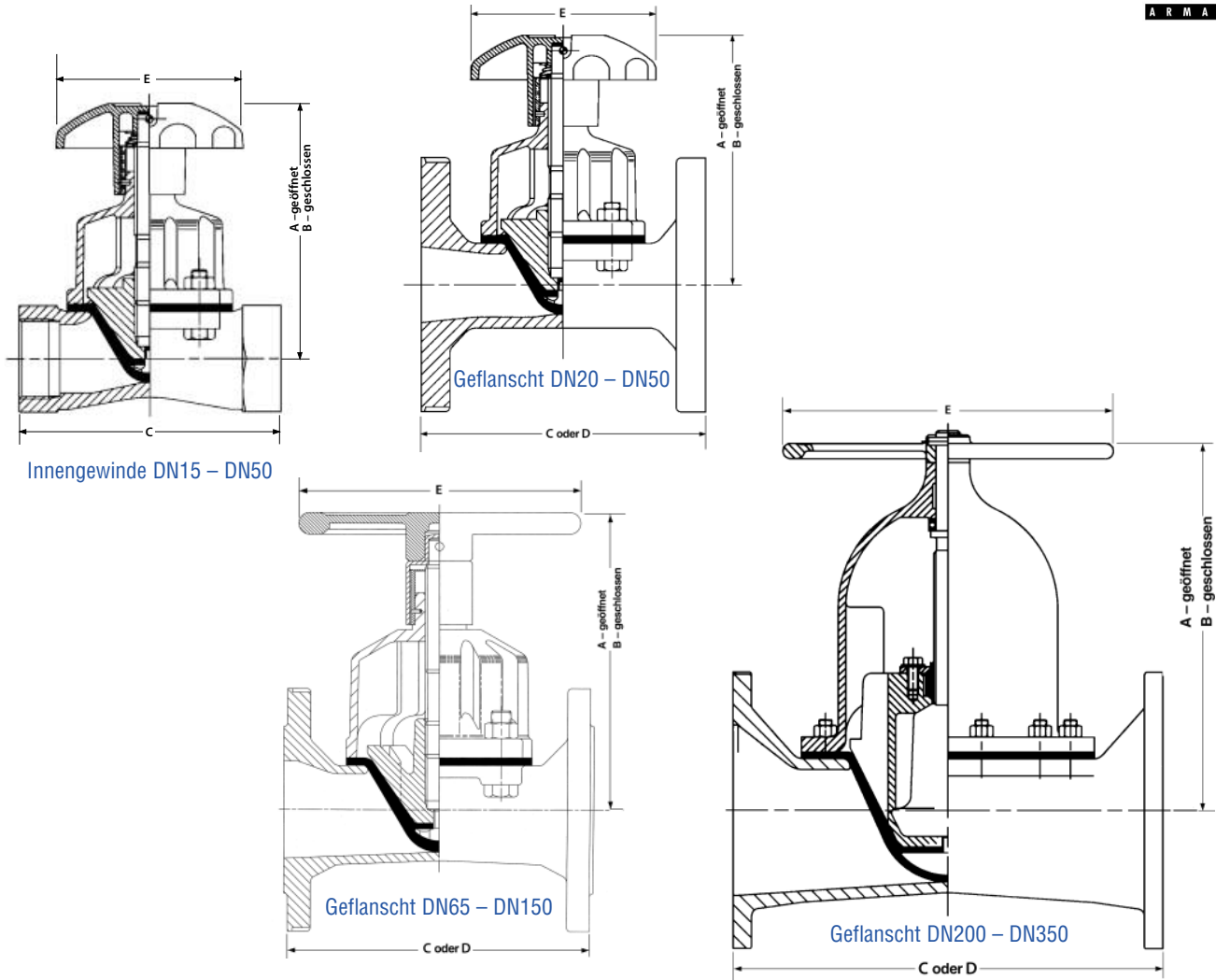
Nennweite (DN) Maße in mm
